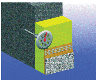
Структура ETICS-системы с полной фиксацией поверхности
