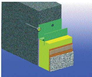
Структура ETICS системы для закрепления направляющих без внешнего крепления
